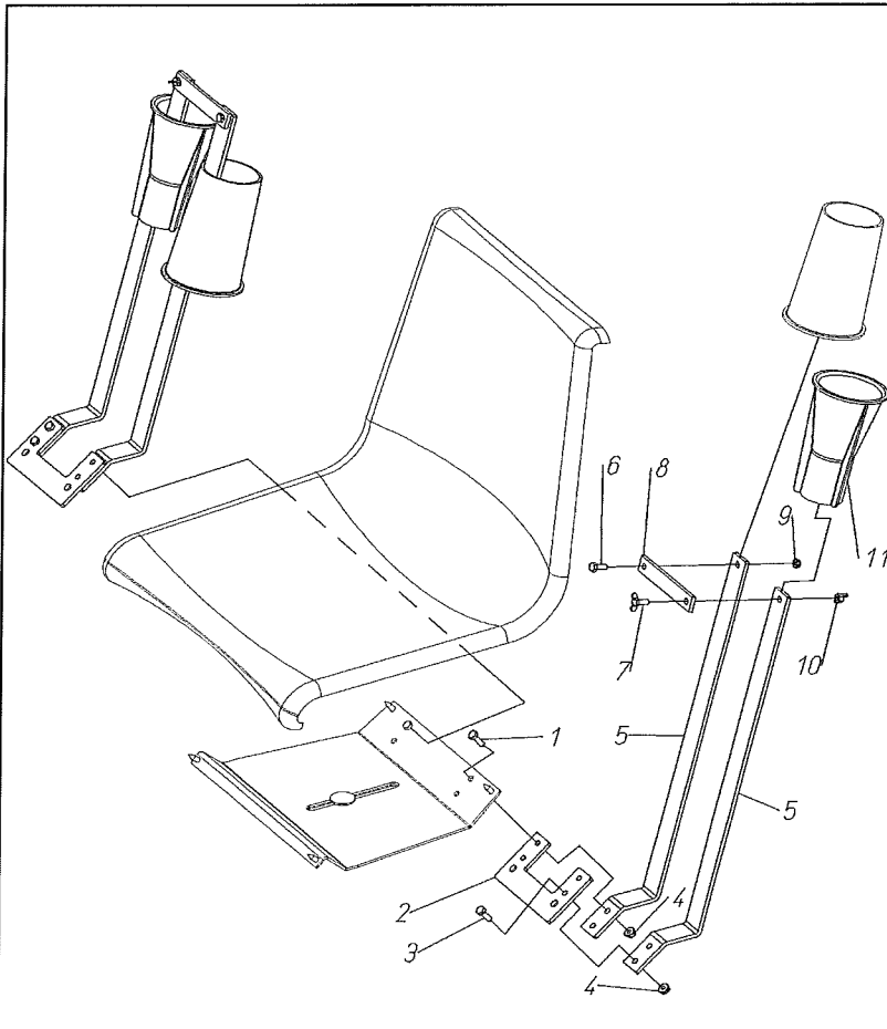
510093-SEDILE IN PLASTICA CON RIDUZIONI
